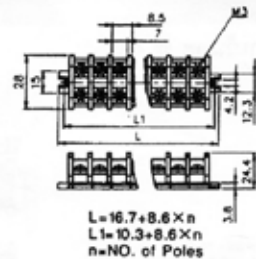
TBC-10H ฝาข้าง (END PLATE) @ 7.-
