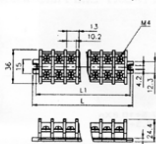
TBC-30H ฝาข้าง (END PLATE) @ 8.-
