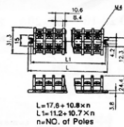
TBC-20H ฝาข้าง (END PLATE) @ 7.-
