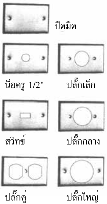
F.S. COVER PLATES SINGLE GANG ฝาปิด เอฟ. เอส. บ็อกซ์ ซิงเกิ้ล แก๊งค์
