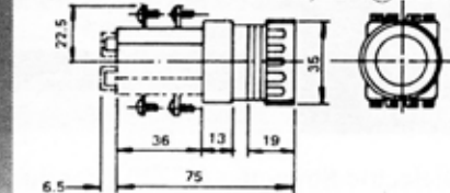
TBW-301 Ø30 mm สวิตช์กดกันน้ำ
